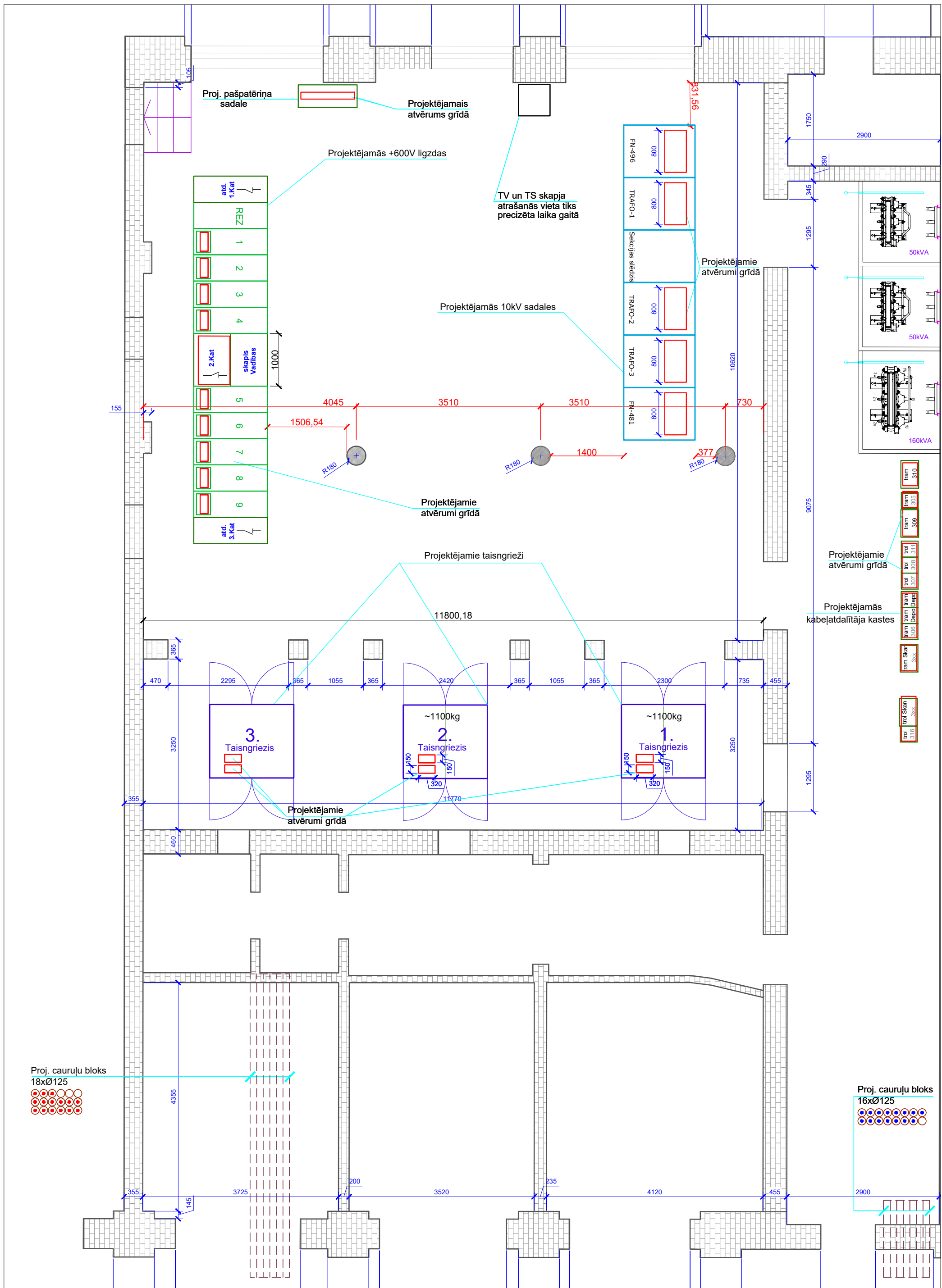
3. Vilces apakšstacija Jauno iekārtu izvietojums
