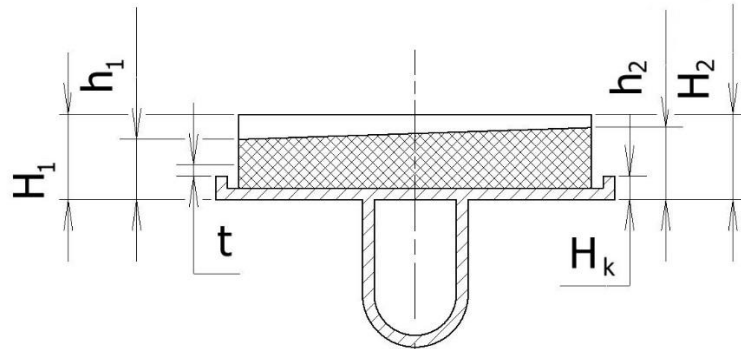
Attēls Nr.2. Pantogrāfa ieliktna mērījumu metode.
