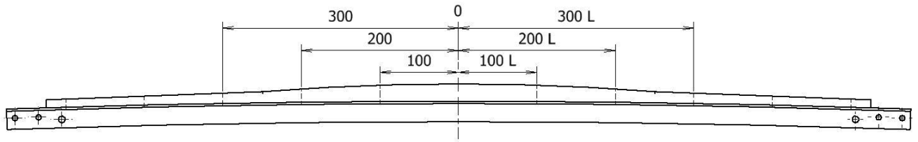
Attēls Nr.1. Pantogrāfa ieliktna mērījumu punkti.
