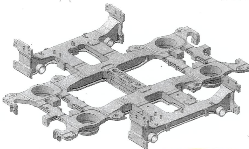
Рама внутренней моторной тележки (B, C или B, C, D)
