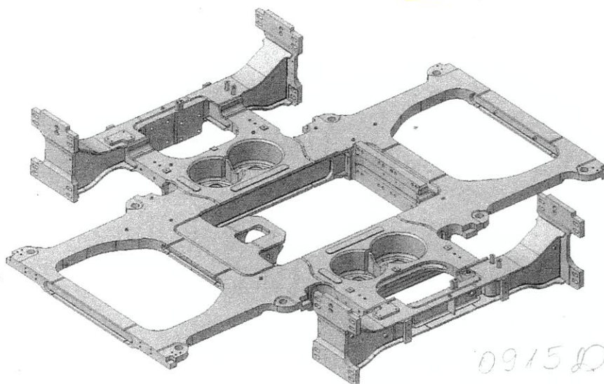
Рама внутренней моторной тележки (B, C или B, C, D)
